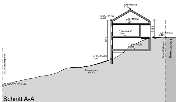
Schnitt A-A
