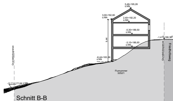
Schnitt B-B
