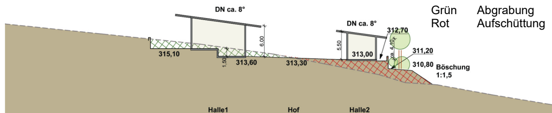
Systemschnitt unmaßstäblich
